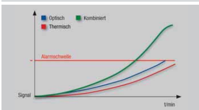
Ansprechverhalten IQ8Quad OT-Melder bei TF 4
