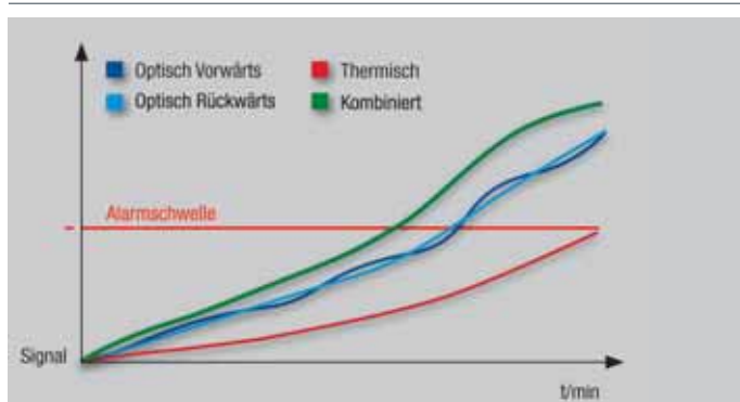
Ansprechverhalten IQ8Quad O 2 T-Melder bei TF 5
